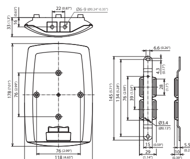
Maßbild
