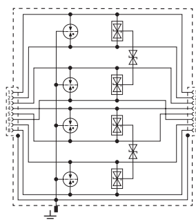
Prinzipschaltbild
